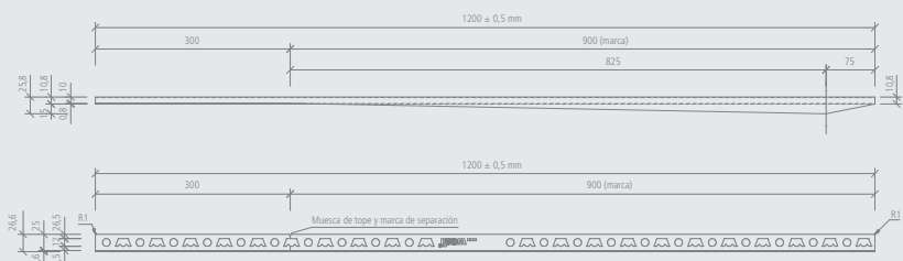
Dibujo técnico Fundo Riolito Perfil, versión izquierdo
