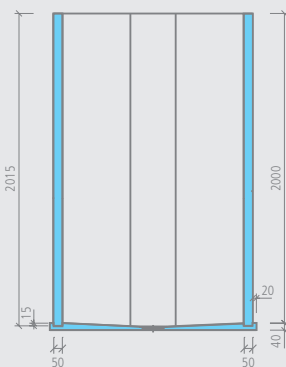
Fundo Trollo libero , ducha de diseño
