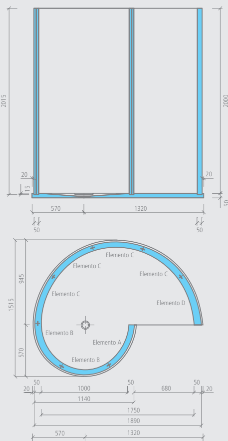
Fundo Nautilo, ducha de diseño
