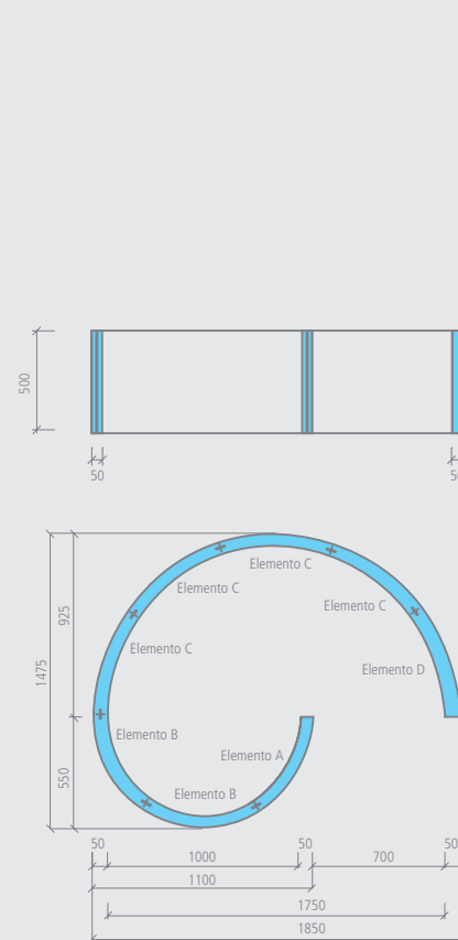
Fundo Nautilo, elemento regulador de altura
