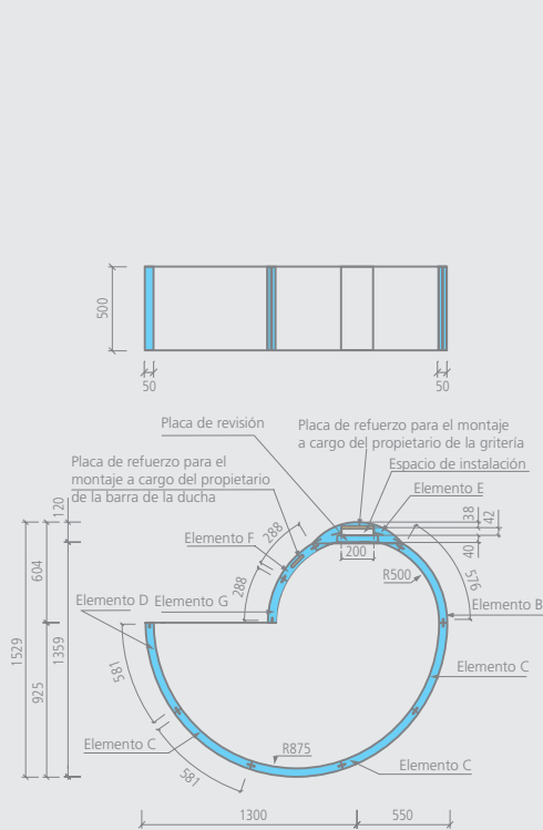
Fundo Nautilo libero , elemento regulador de altura
