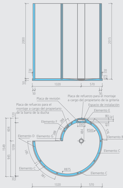
Fundo Nautilo libero , ducha de diseño
