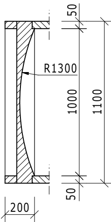
Schnitt B-B
