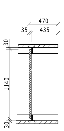
Ansicht Holz-Sitzbank
