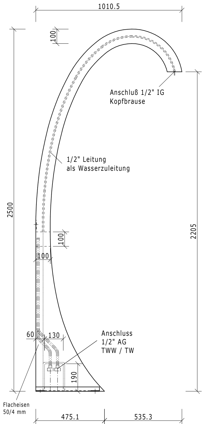
Seitenansicht
