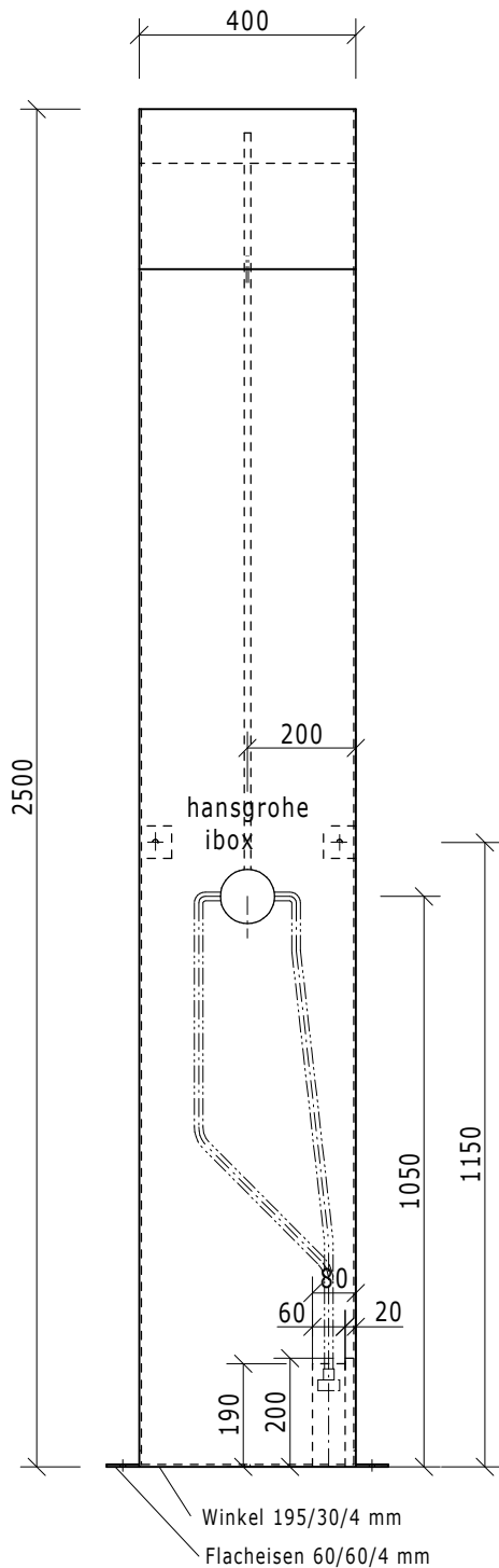
Ansicht
