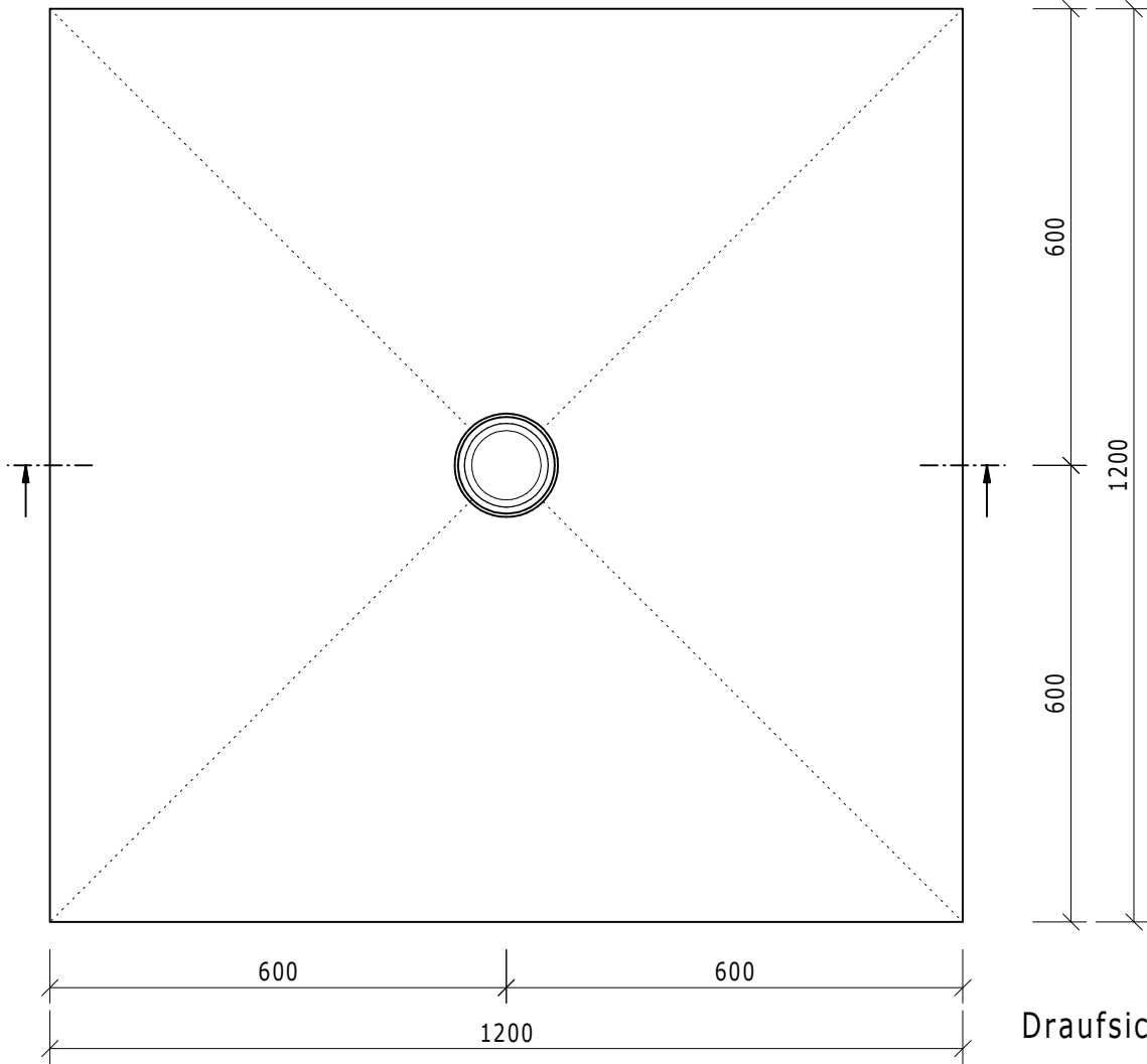
Schnitt
